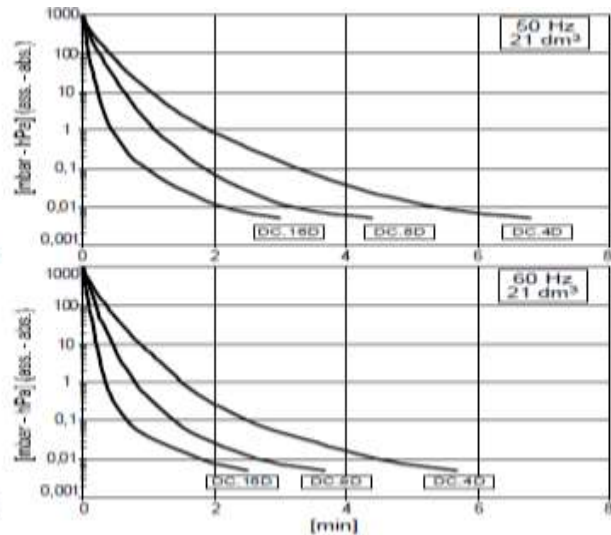
NOTA: Grafico com referência à pressão de aspiração e temperatura de 20°C (tolerância ±10%)
